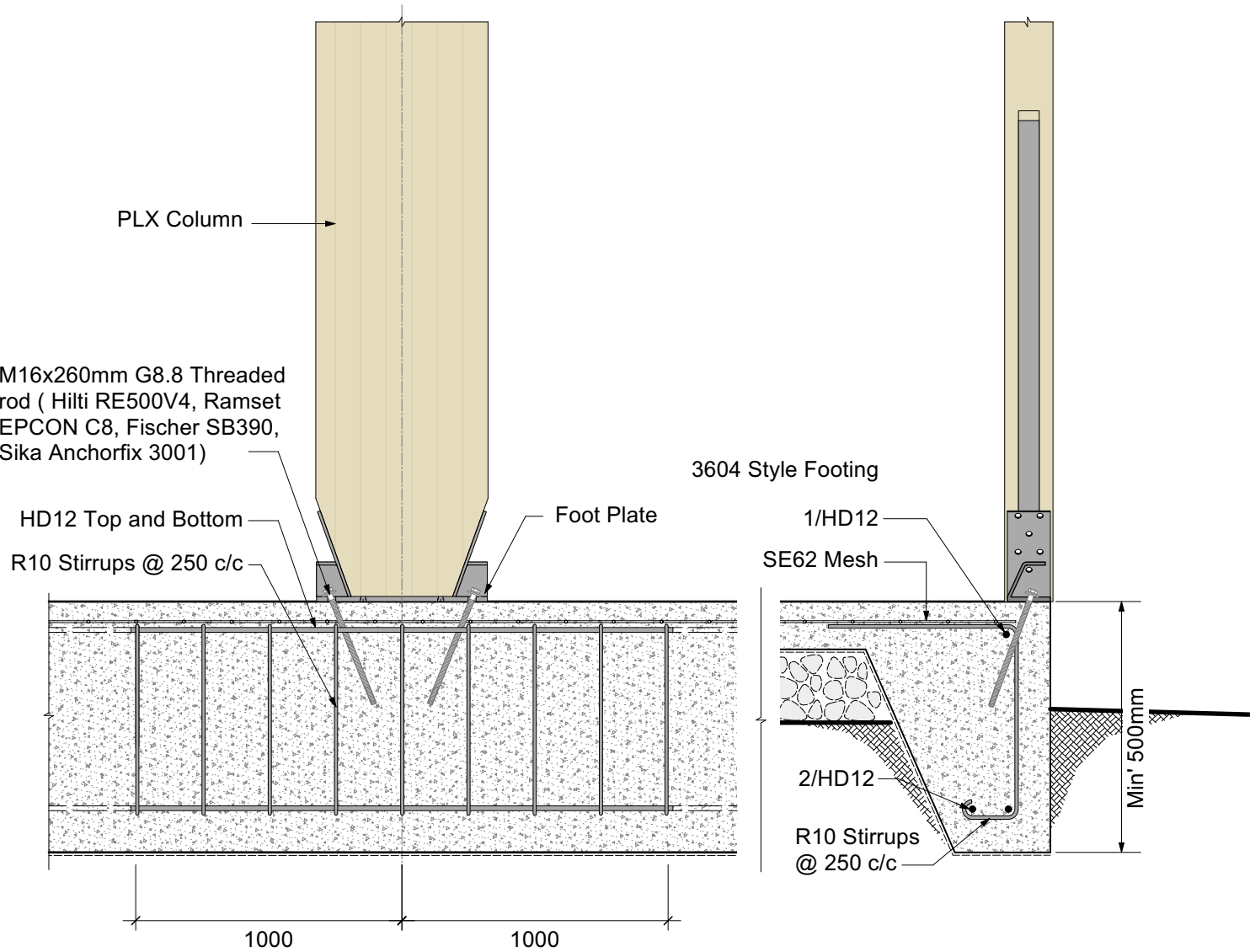
LONGITUDINAL SECTION
